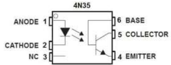
Fig.3. 4N35 Optocoupler pin layout
